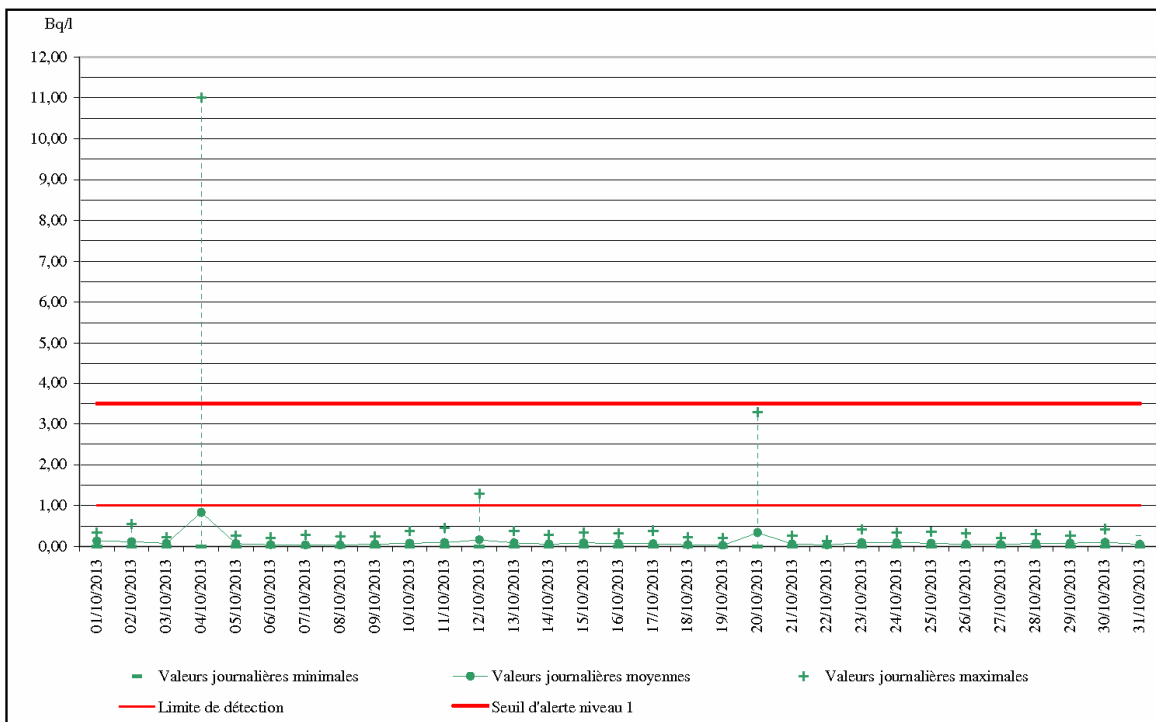
Evolution des activités volumiques de la voie « iode 131 » - octobre 2013
